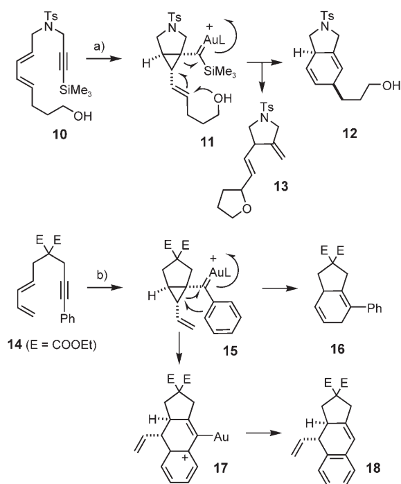
Scheme 2. a) [(Ph 3 P)AuCl] (5 mol %), AgSbF 6 (5 mol %), CH 2 Cl 2 , 12 (68 %), 13 (15 %); b) [(Ph 3 P)AuCl] (5 mol %), AgSbF 6 (5 mol %), CH 2 Cl 2 , 78 % ( 16/18 ca. 3:4).
